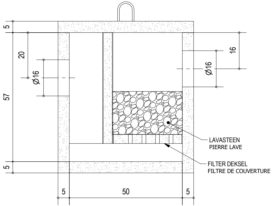
A-A VOORAANZICHT VUE DE FACE
